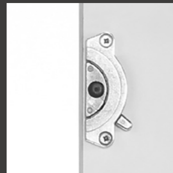
Plattenverbinder table top connector
