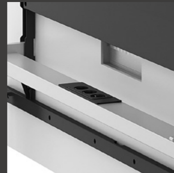
Einbaubox in Rahmen des Konferenztischgestells mit Klappe in der Tischplatte (tischmitten) Installation box in the conference-table frame with table top flap (table centre)
