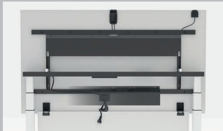
// Kabelmanagement ohne/mit horizontalem Kabelkanal // cable management without/with horizontal cable duct
