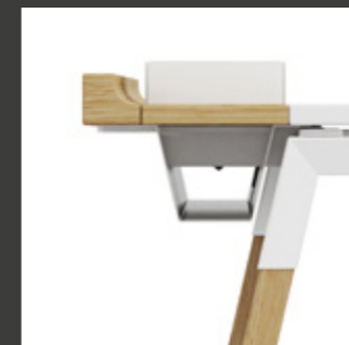
Abschlussleiste und HomeLine Kabelwanne End profile and cable tray
